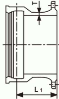
■ 短管1號 Flanged Socket
