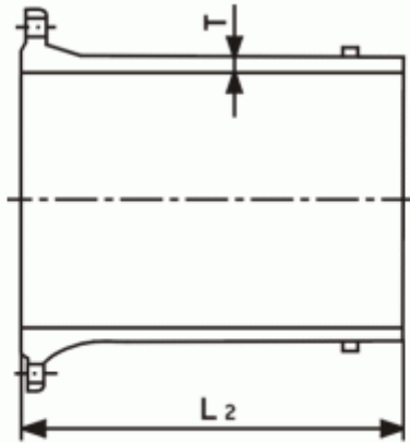
■ 短管2號 Flanged Spigot
